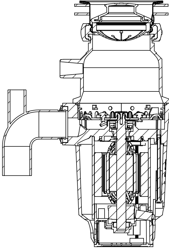
KESİT A-A ÖLÇEK 1 : 3
