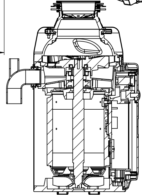
KESİT A-A ÖLÇEK 1 : 6
