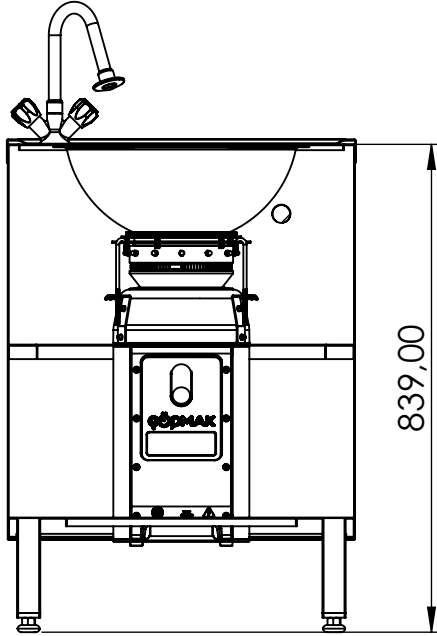
KESİT A-A ÖLÇEK 1 : 13
