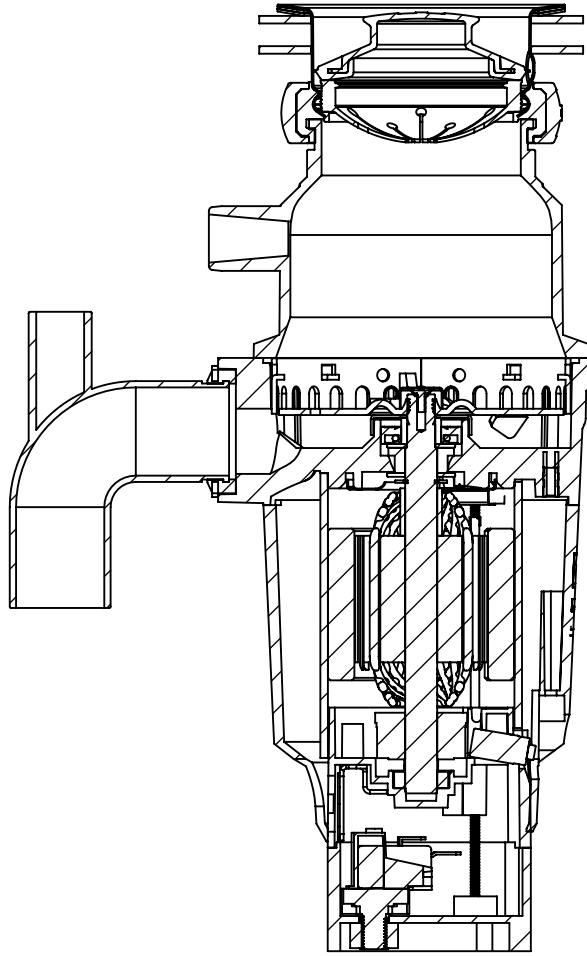
KESİT A-A ÖLÇEK 1 : 3
